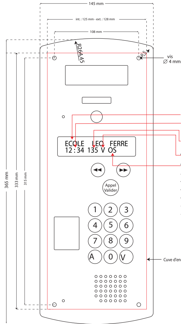
Cotes de la platine d'interphone
