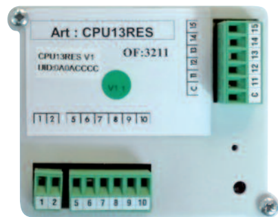
Lecteur CléLib lecteur de badges de proximité réf. : D201JPROX
